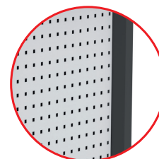
Perforations latérales carré de 10 au pas de 38 pour accroche outillage
