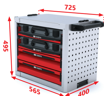
Présentation des blocs ISIBLOC Réf. IB52-2T et IB54-3T empilés
