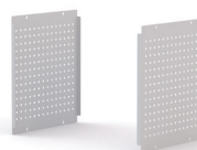
2 panneaux perforés latéraux 660 x 575 - 3.1 kg Réf. PPL-E
