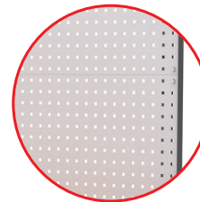
Perforations carré de 10 au pas de 38 pour accroche outillage
